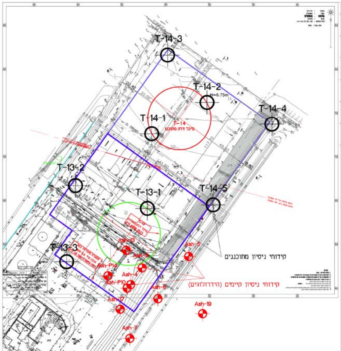
איור 1 – תוכנית העמדה כללית ומיקום קידוחי ניסיון.
